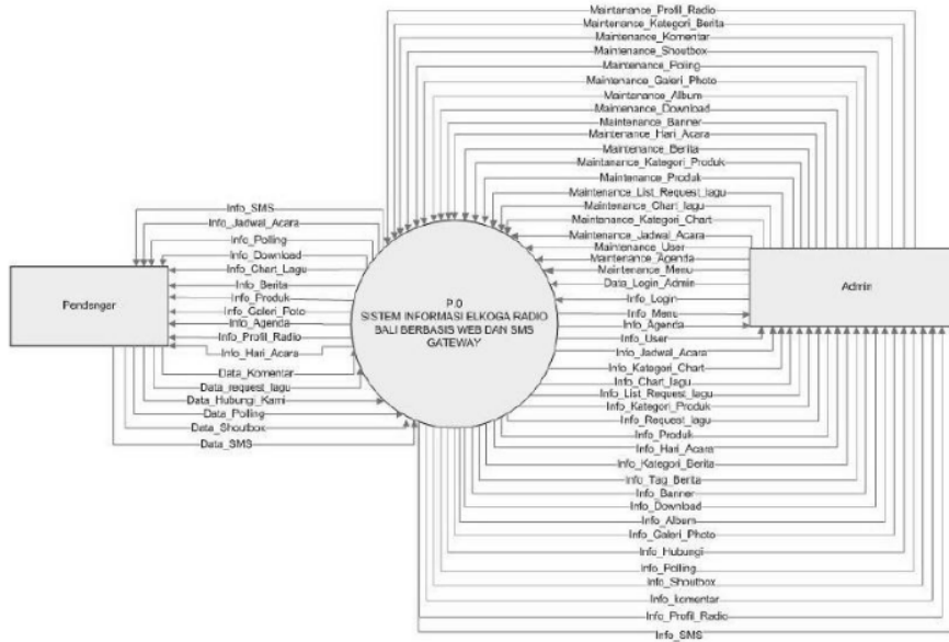
Gambar 2. Diagram Konteks Sistem Informasi Elkoga Radio Bali
