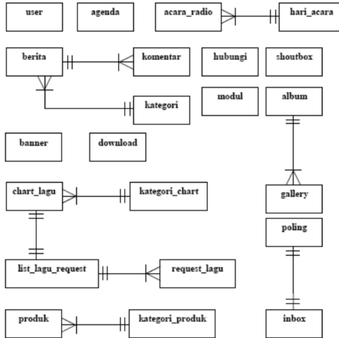
Gambar 4. ERD Sistem Informas Elkoga Radio Bali
