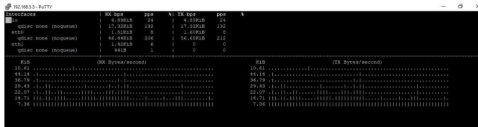
Gambar 7. Trafik monitoring dengan BMON pada saat ada 3 client yang terhubung.
