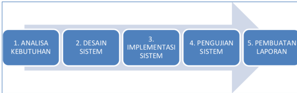
Gambar 1. Tahapan Penelitian
